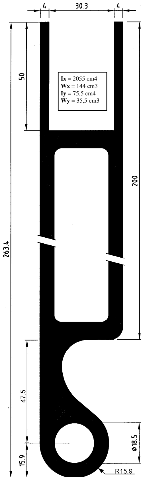
FL 26481 10,09 kg/m code 418317 7,50 m
