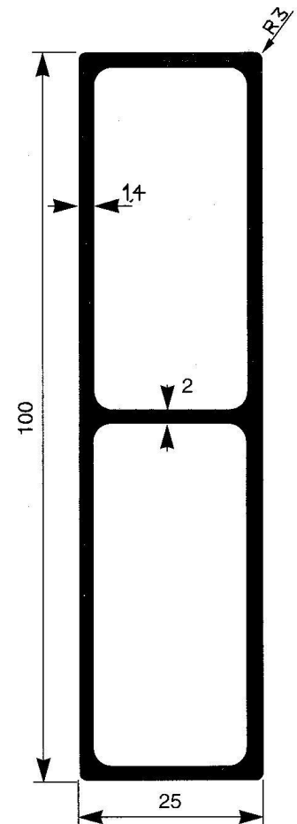
AL 28014 1,1 kg/m code *
