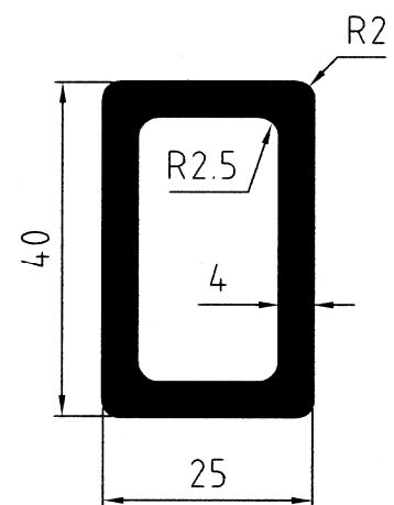
AL 10832 1,27 kg/m code 1100495 7,60 m
