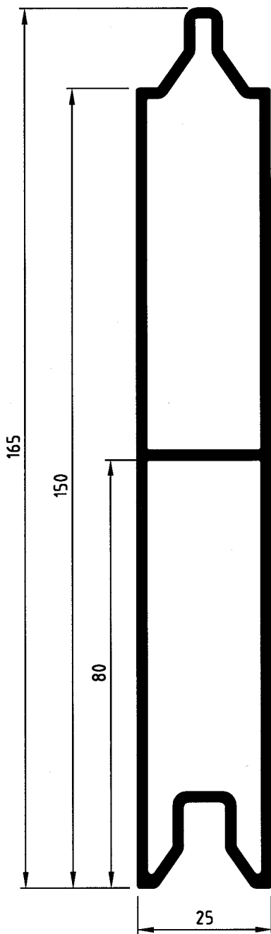
DC 07970 2,00 kg/m code 1100232 3,24 m 403514 6,65 m 903055 7,50 m
