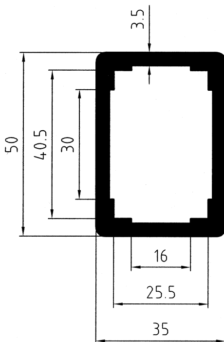
DC 07686 1,61 kg/m code 1100095 7,60 m
