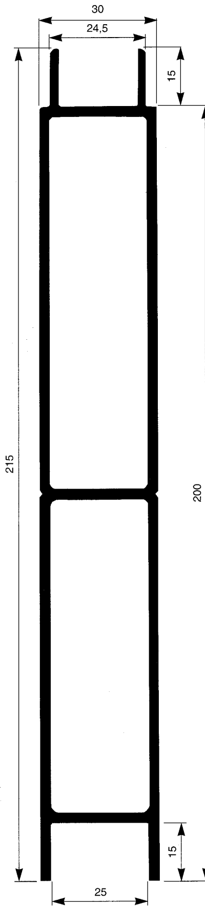
FL 20064 2,94 kg/m code 371016 7,35 m
