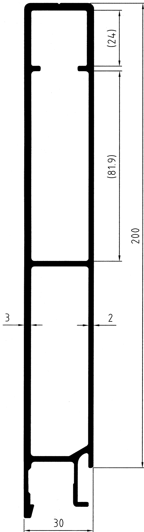
DC 11924 3,49 kg/m code 1102271 7,50 m
