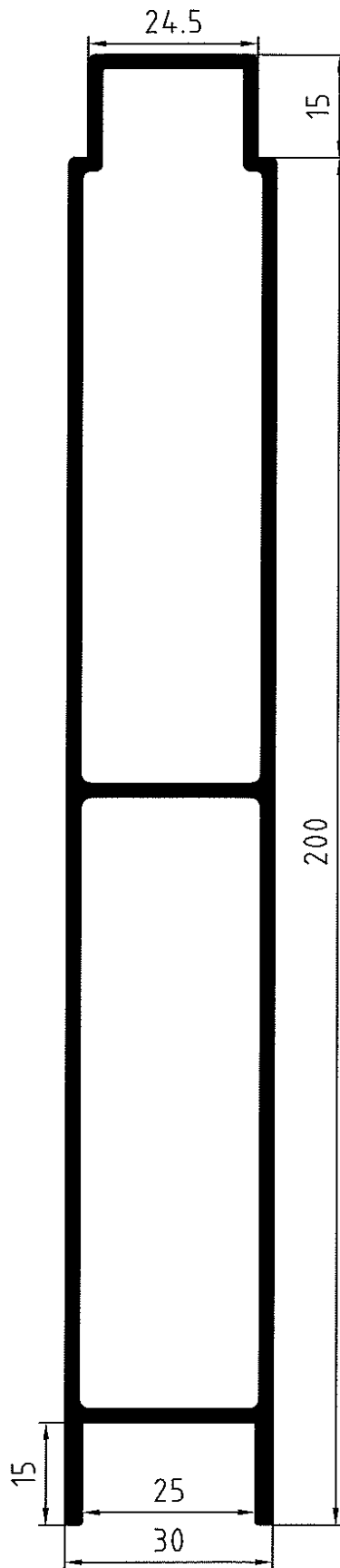
AL 03349 2,79 kg/m code 1104726 6,20 m 1104725 7,00 m
