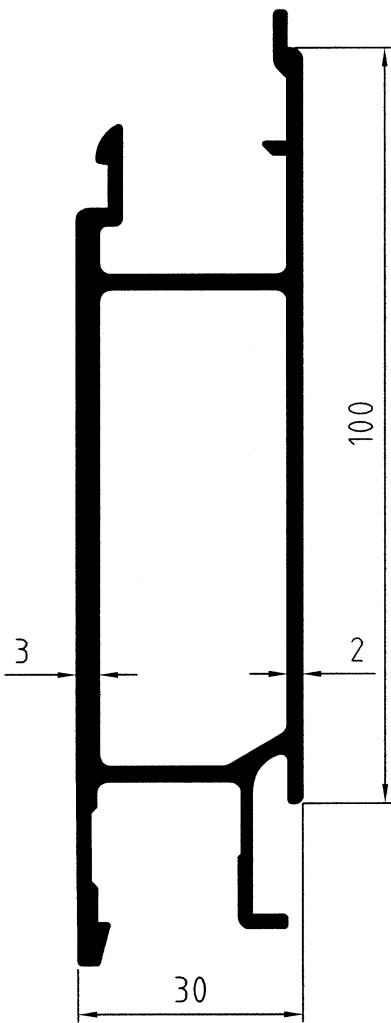
DC 12008 1,90 kg/m code 1102397 7,50 m
