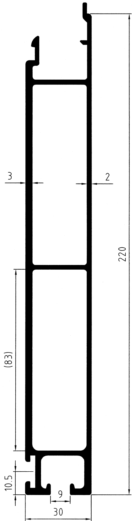
DC 11925 3,57 kg/m code 1102270 7,50 m
