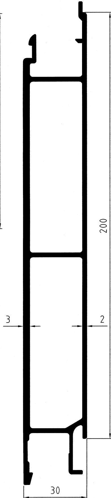
DC 11448 3,40 kg/m code 1101127 7,50 m
