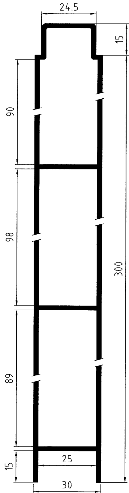
AL 43636 3,91 kg/m Code 1104590 6,20 m 1104589 7 m
