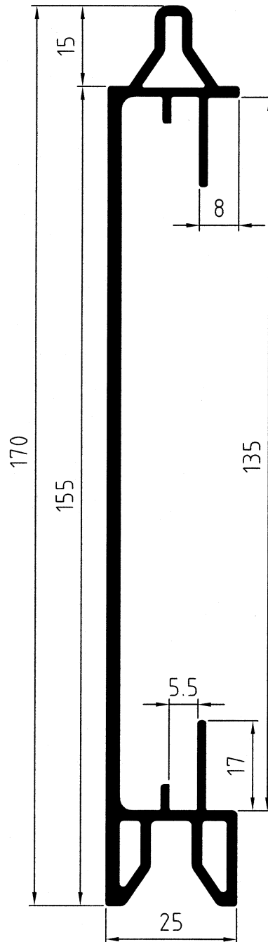
AL 27796 1,90 kg/m code 1102399 7,50 m
