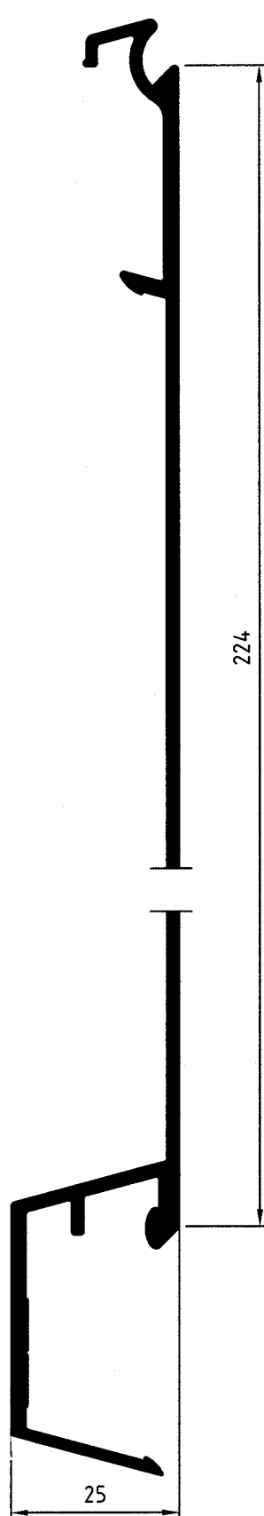
DC 07908 2,10 kg/m Code 1100133 5,60 m 1100171 7,50 m
