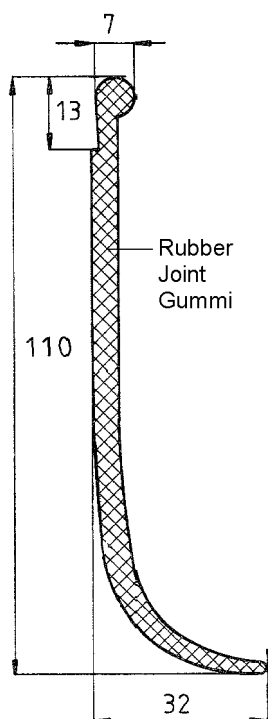
AN 621 0,87 kg/m Code 642303 28,00 m
