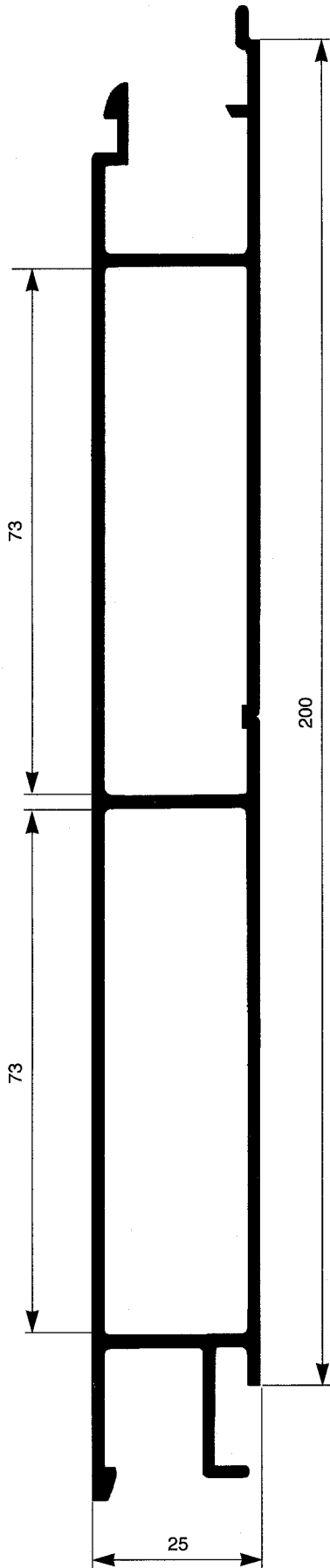
DC 10160 2,30 kg/m Code 1100173 7,50 m
