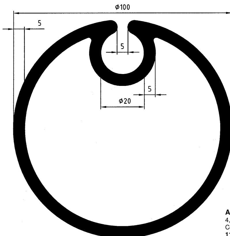
AN 621 0,87 kg/m Code 642303 28,00 m
