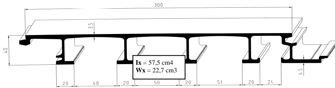
AL 12368 6,61 kg/m code 406817 7,50 m
