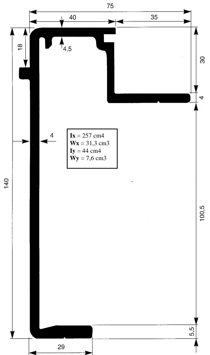
CH 52362 3,02 kg/m code 390416 7,30 m
