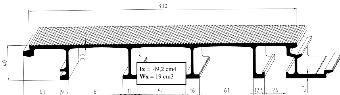
AL 12369 6,07 kg/m code 406917 7,50 m
