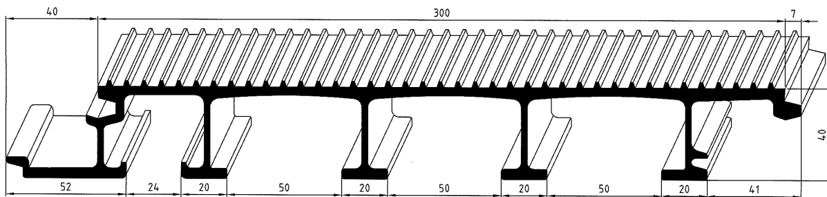
AL 45330 7,15 kg/m code 1104901 7,50m
