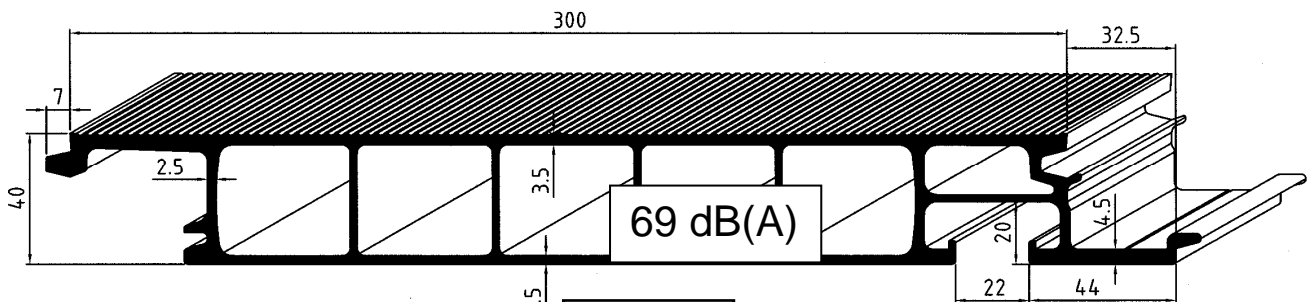
CH 56807 7,76 kg/m code 404017 7,50 m
